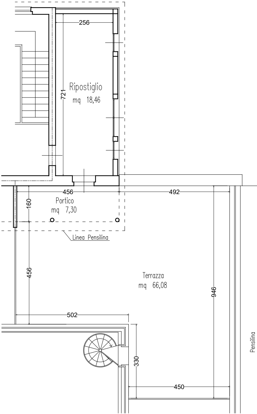
PIANO SECONDO
